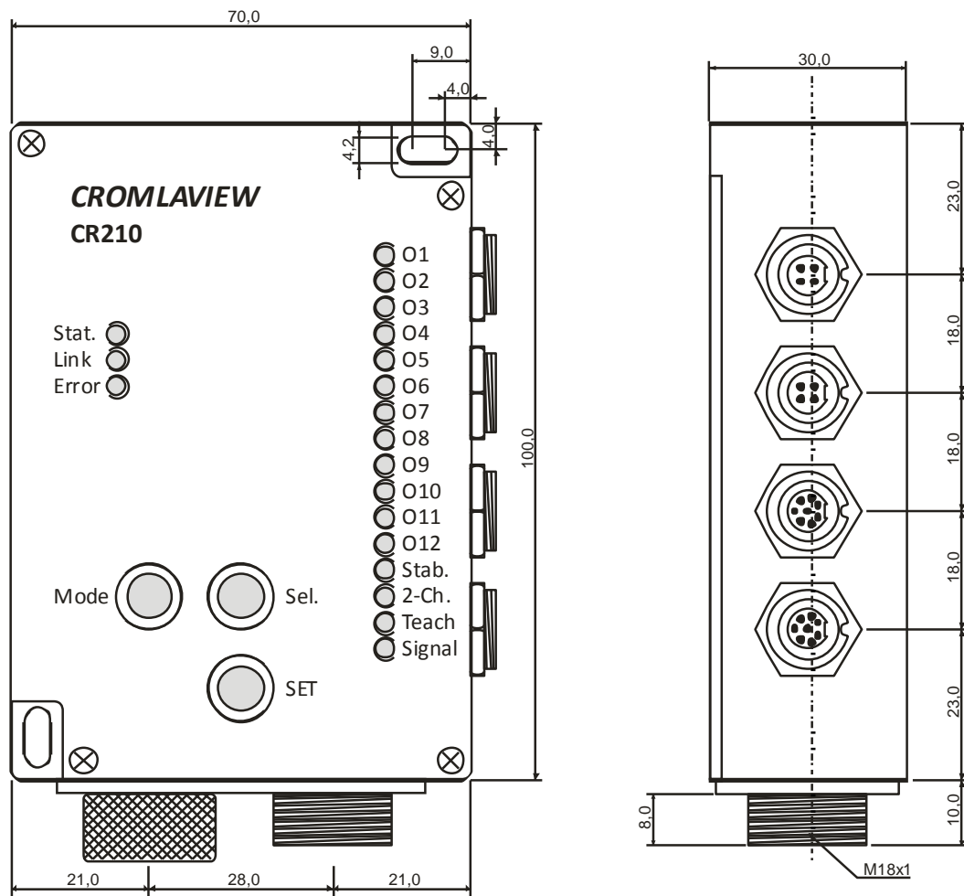
Abbildung 4 : CR210 mit eingebauter Stellvorrichtung für die Driftstabilisierung CROMLASTAB®
