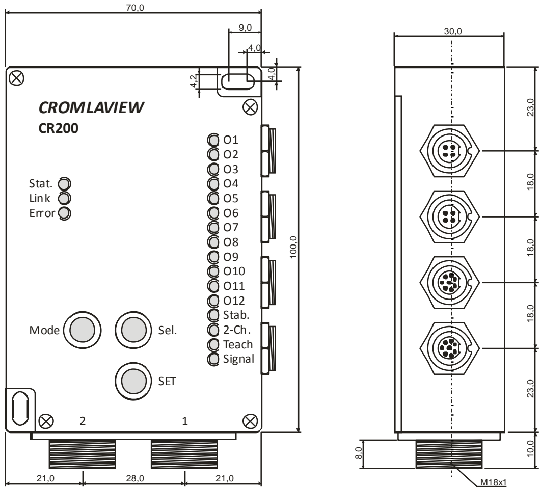
Abbildung 3 : CR200 zum Anschluss von zwei getrennten Lichtleitern
